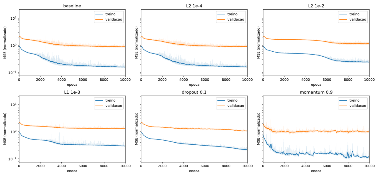
Figura 3: Evolução do treinamento para o baseline e configurações representativas de cada componente.
